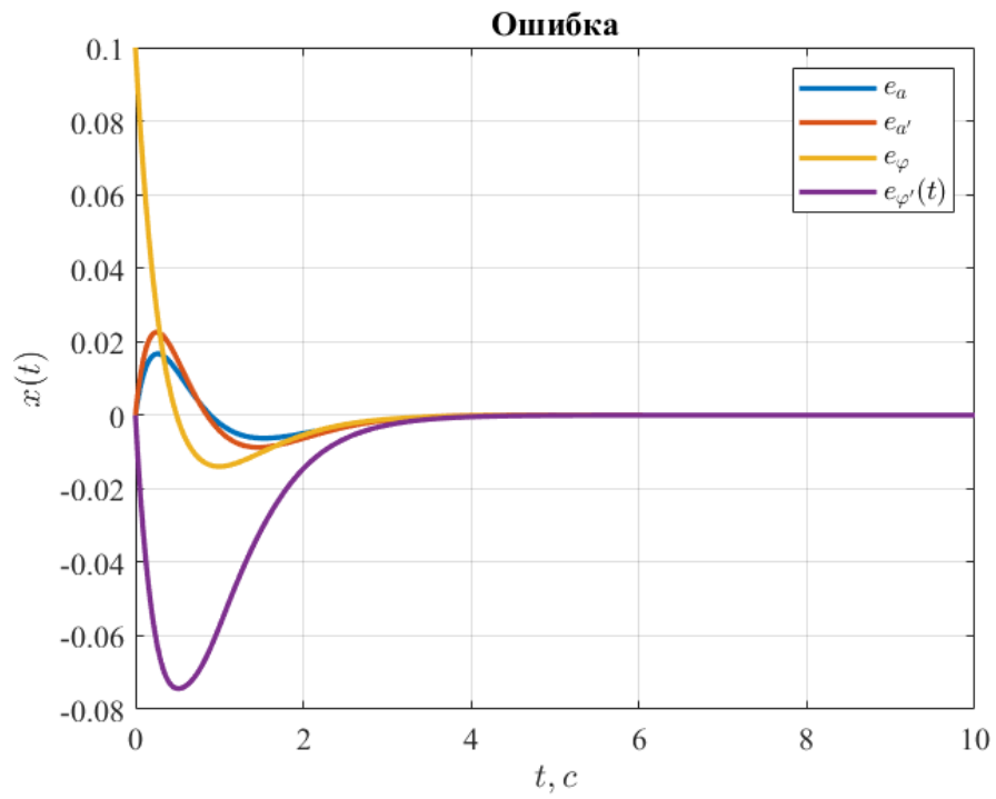
Рисунок 30. Ошибка наблюдателя – второй случай.
