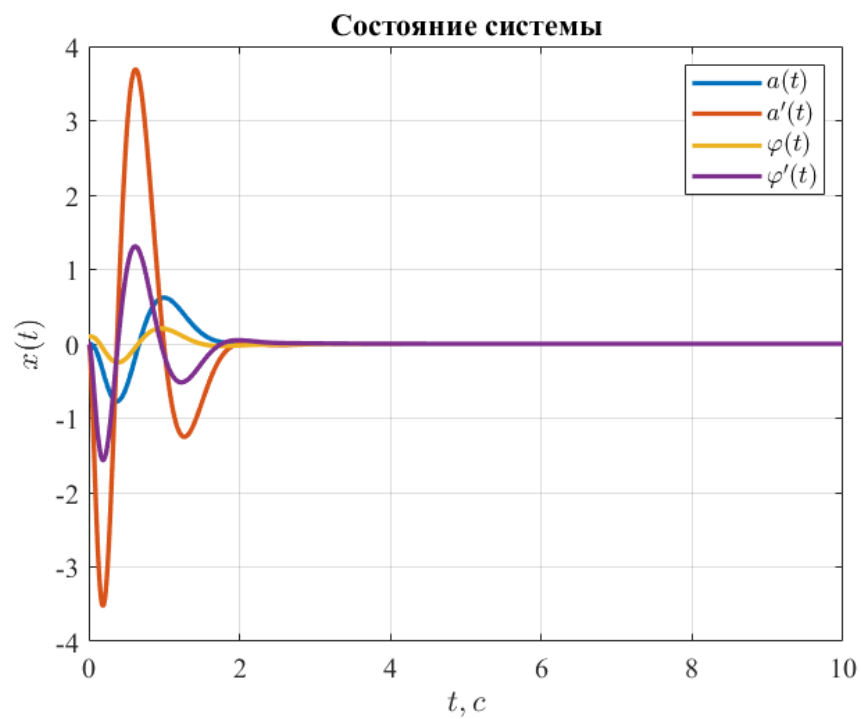
Рисунок 54. Состояние системы – третий случай.
