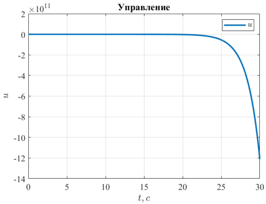
Рисунок 67. Управление нелинейной модели.
